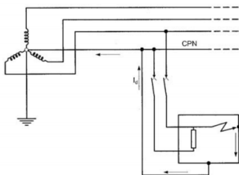
Ilustración 27: Conexión TN-C en estrella
