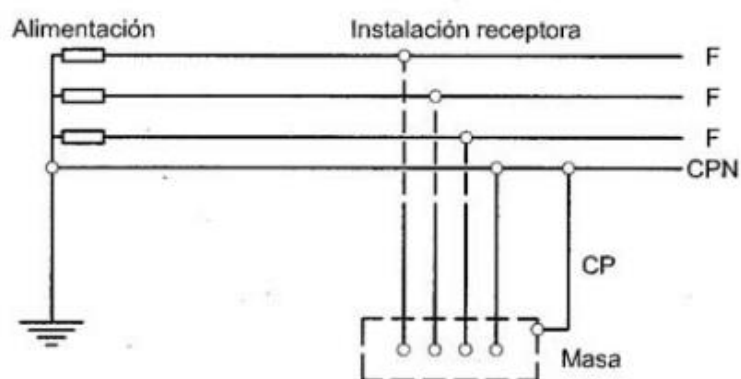
Ilustración 25: Esquema TN-C.
