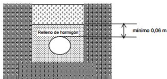
Ilustración 48: Tubo con recubrimiento de hormigón, resistencia a la compresión mínima 250 N
