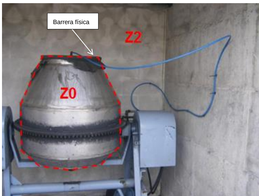
Ilustración 3: Detalle de bombo de mezcla cerrado
