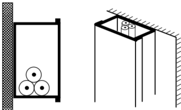
Ilustración 52: Ejemplo de instalación de conductores unipolares aislados en canal protector superficial
