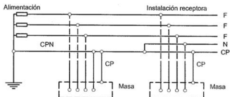
Ilustración 26: Esquema TN-C-S.
