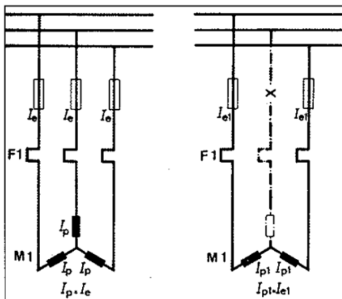
Ilustración 21: Motor de conexión en estrella en funcionamiento normal y en caso de fallo de fase
