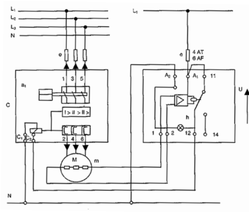
Ilustración 20: Protección por sonda térmica
