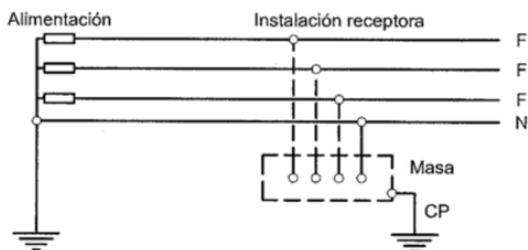
Ilustración 29: Esquema TT
