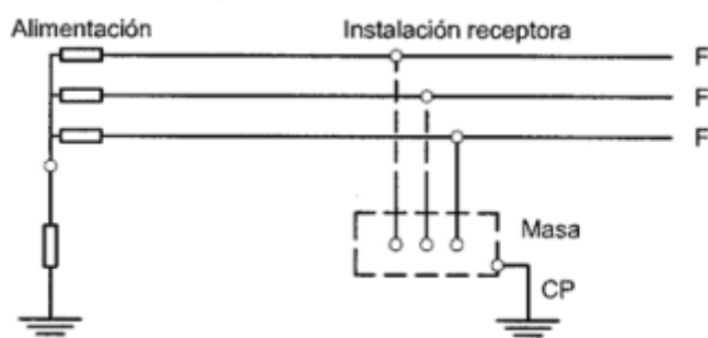
Ilustración 30: Esquema IT
