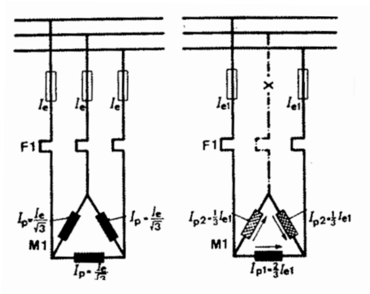
Ilustración 22: Motor de conexión en triángulo en funcionamiento normal y en caso de fallo de clase
