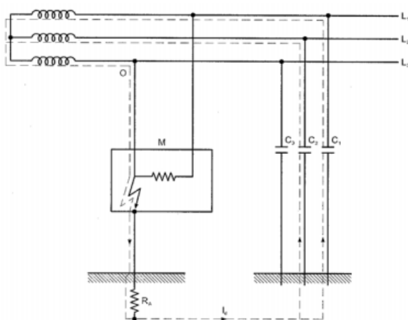
Ilustración 31: Esquema IT aislado de tierra
