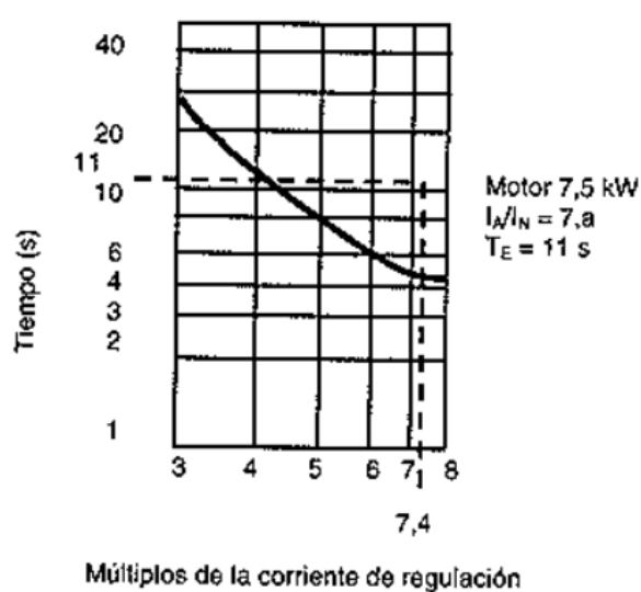
Gráfico 3: Comprobación del relé frente al t_E
