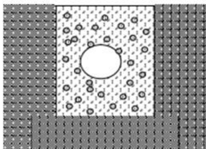
Ilustración 49: Tubos sin recubrimiento en terreno pedregoso , resistencia a la compresión mínima 750 N
