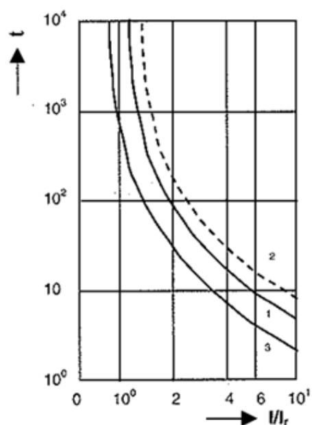
Gráfico 5: Curvas características de disparo de un relé tripolar contra sobrecargas
