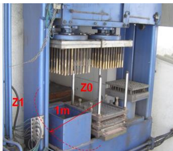
Ilustración 4: Prensa
