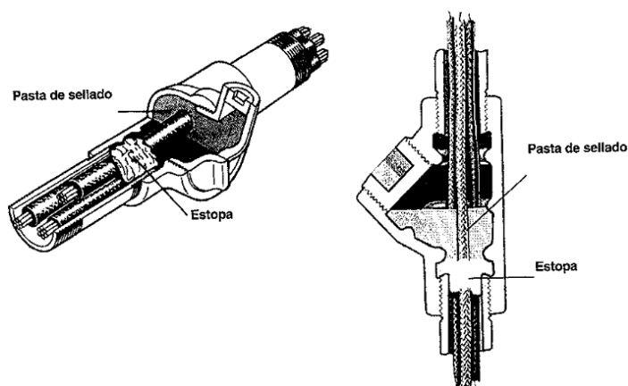
Ilustración 54: Cortafuegos
