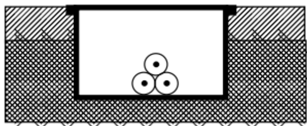
Ilustración 51: Ejemplo de instalación de conductores unipolares aislados en canal protector empotrado en suelo o pared
