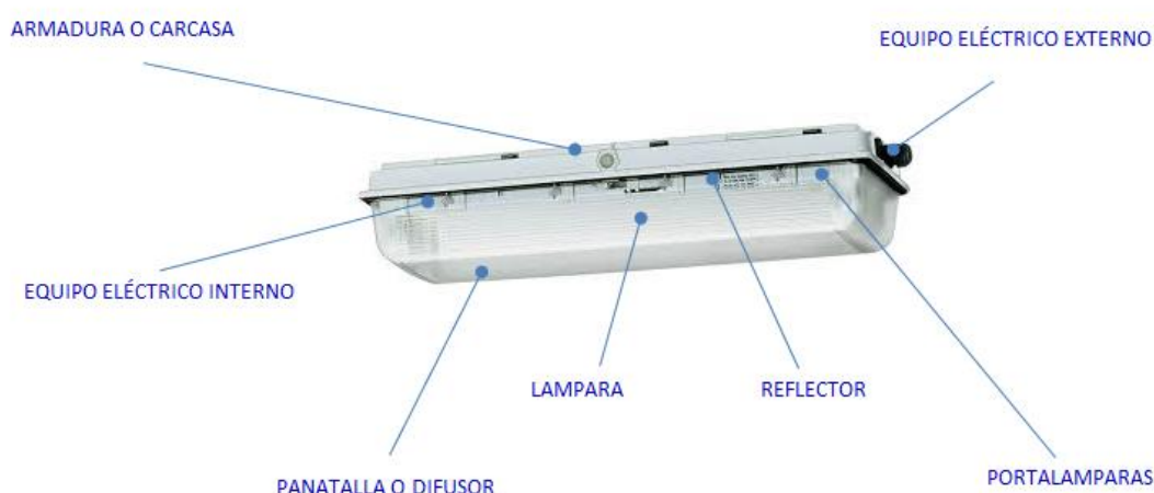
Ilustración 53: Luminaria
