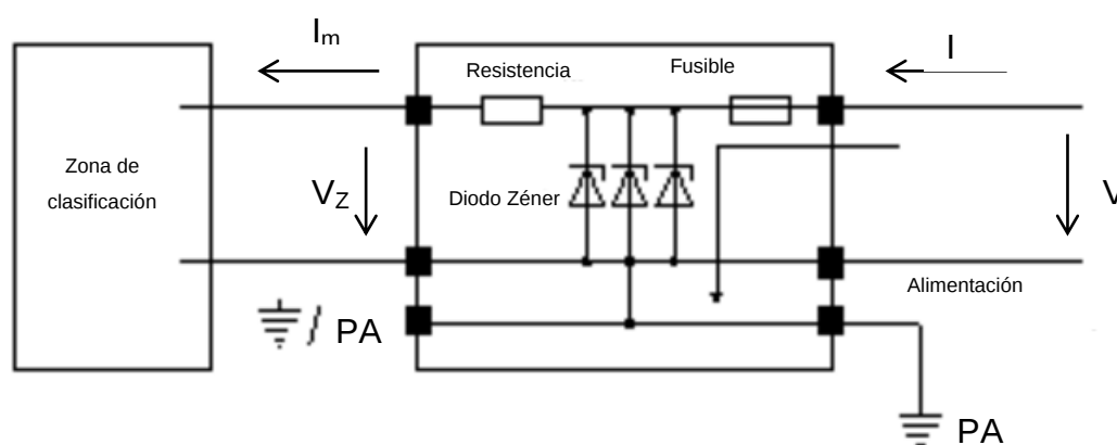
Ilustración 19: Barrera Zéner
