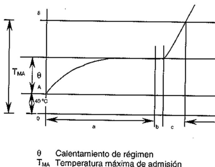
Gráfico 4: Significado del tiempo t_E
