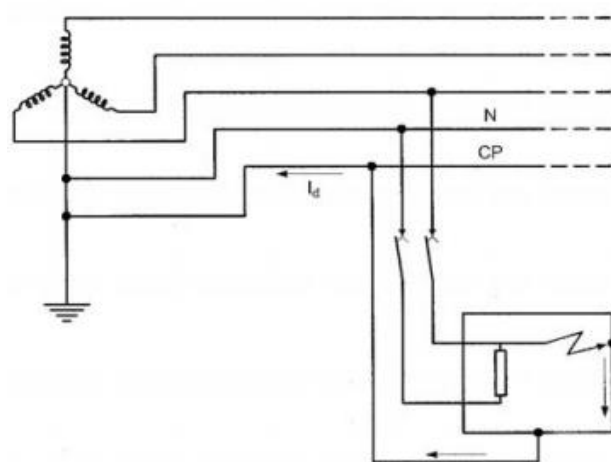
Ilustración 28: Conexión TN-S en estrella
