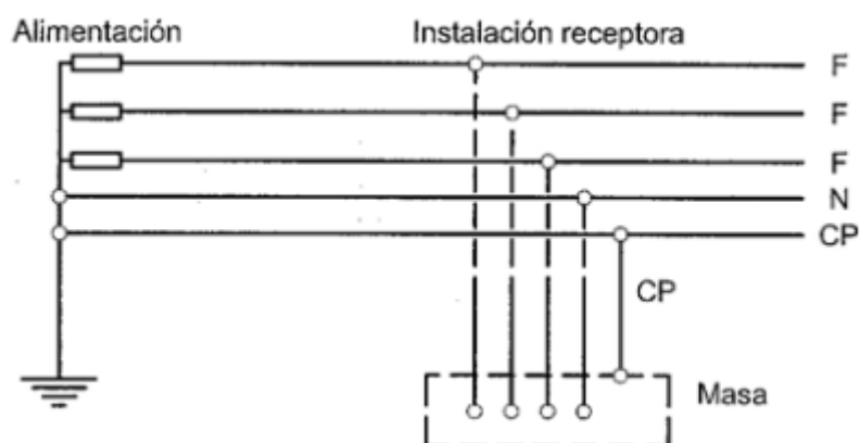
Ilustración 24: Esquema TN-S
